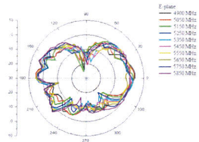
5GHz E-Plane
