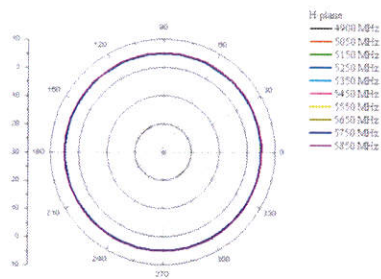
5GHz H-Plane
